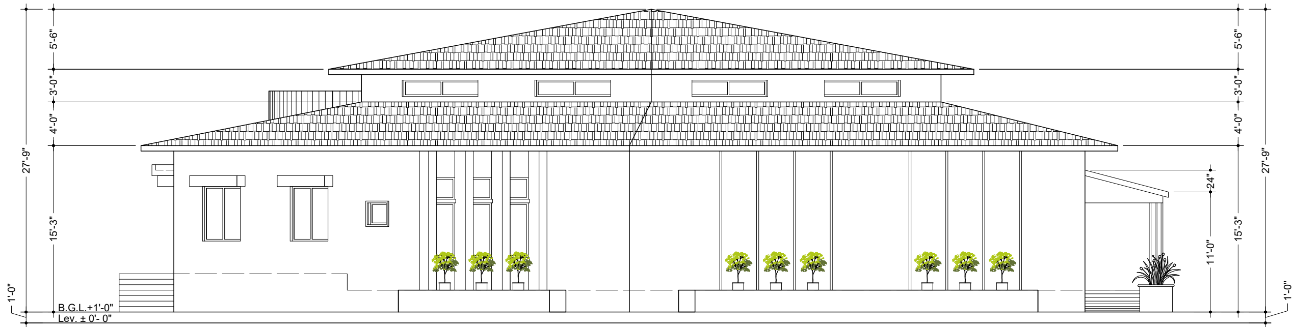
LEFT ELEVATION - 02
