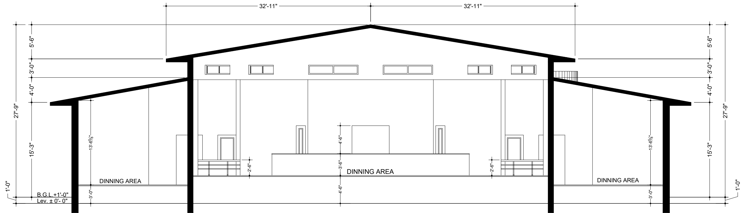
SECTION A-A
