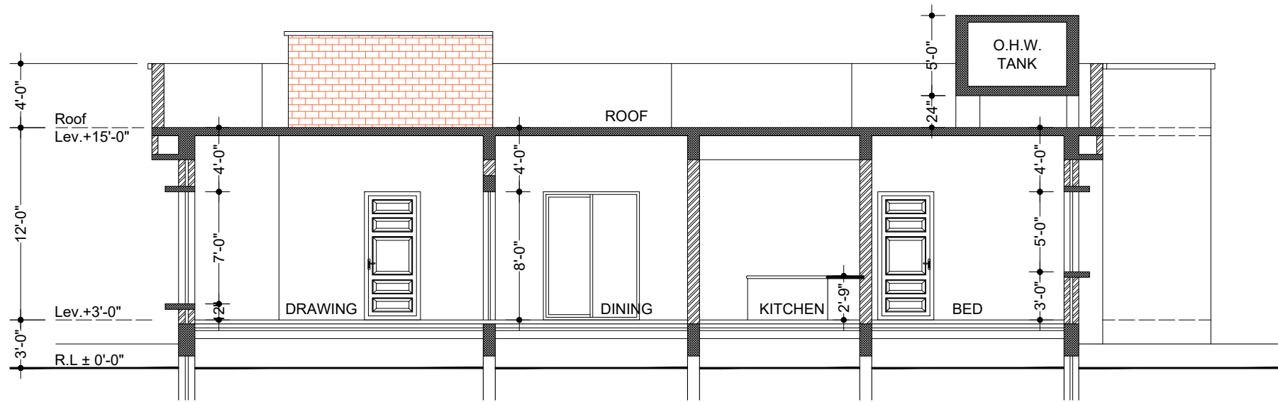
SECTION A-A
