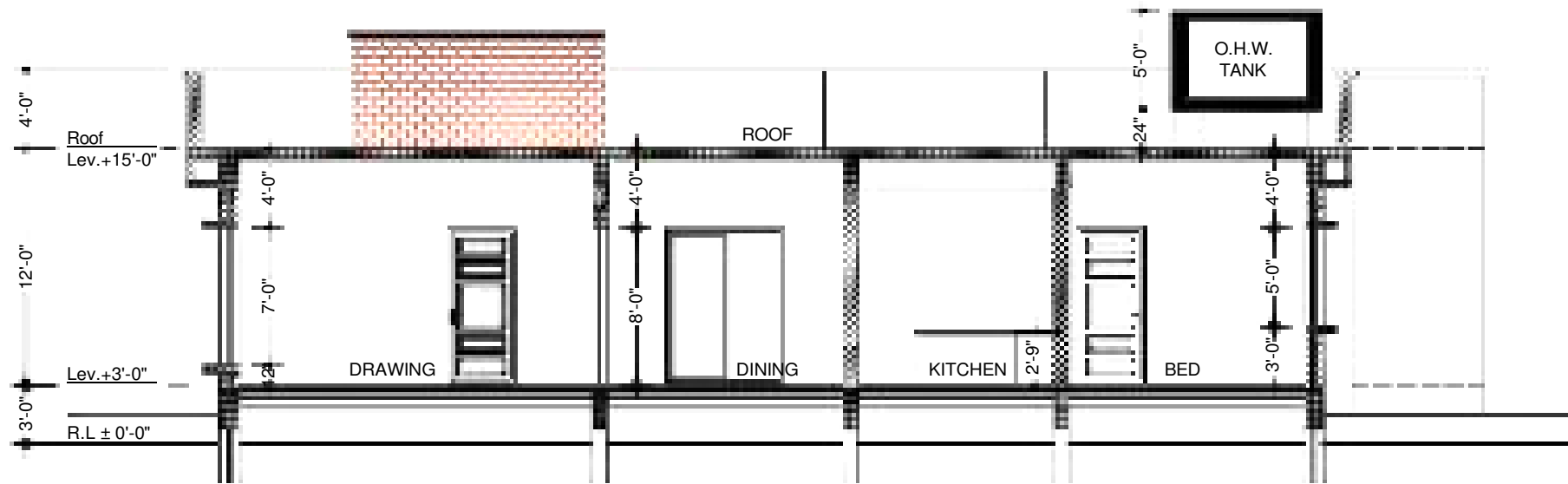
SECTION A-A
