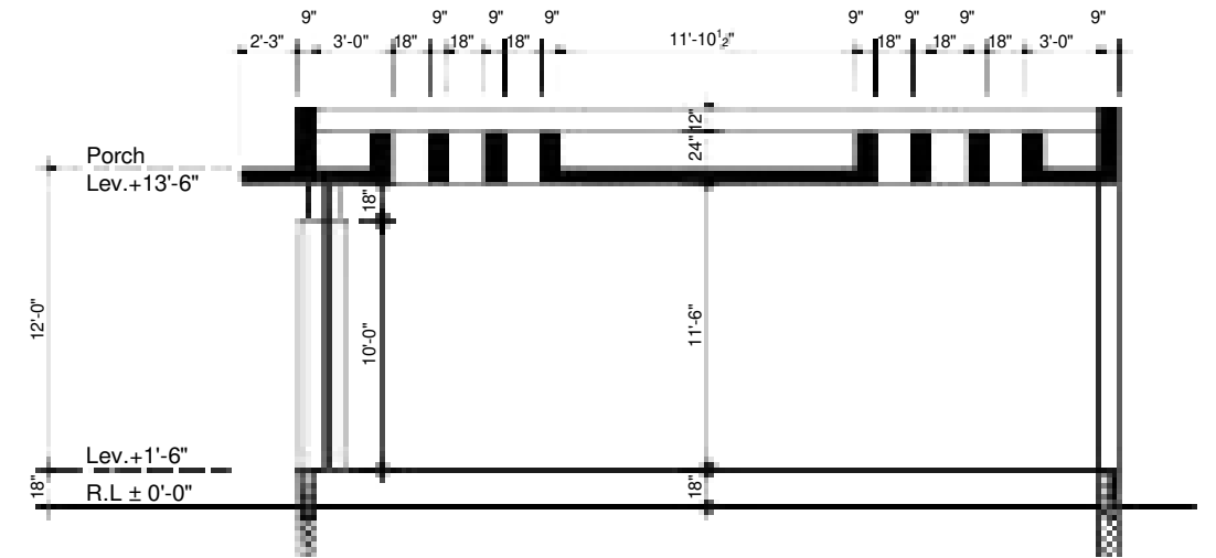
SECTION D-D
