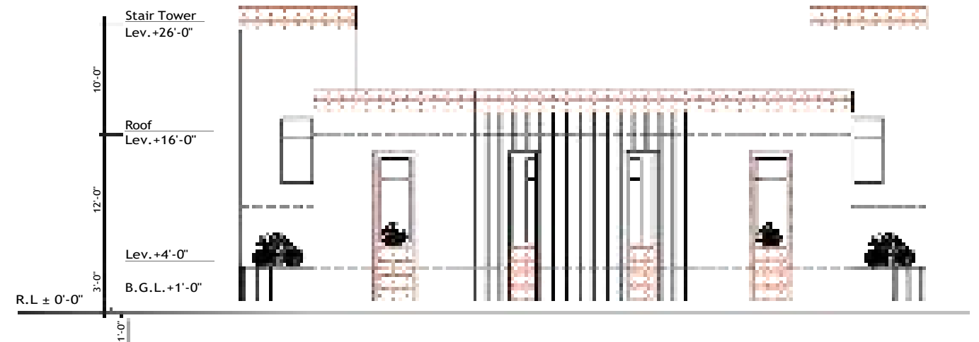
ELEVATION -03
