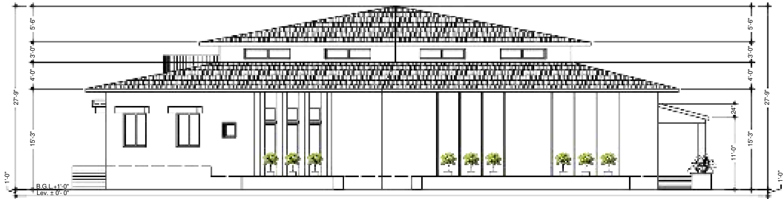
LEFT ELEVATION - 02
