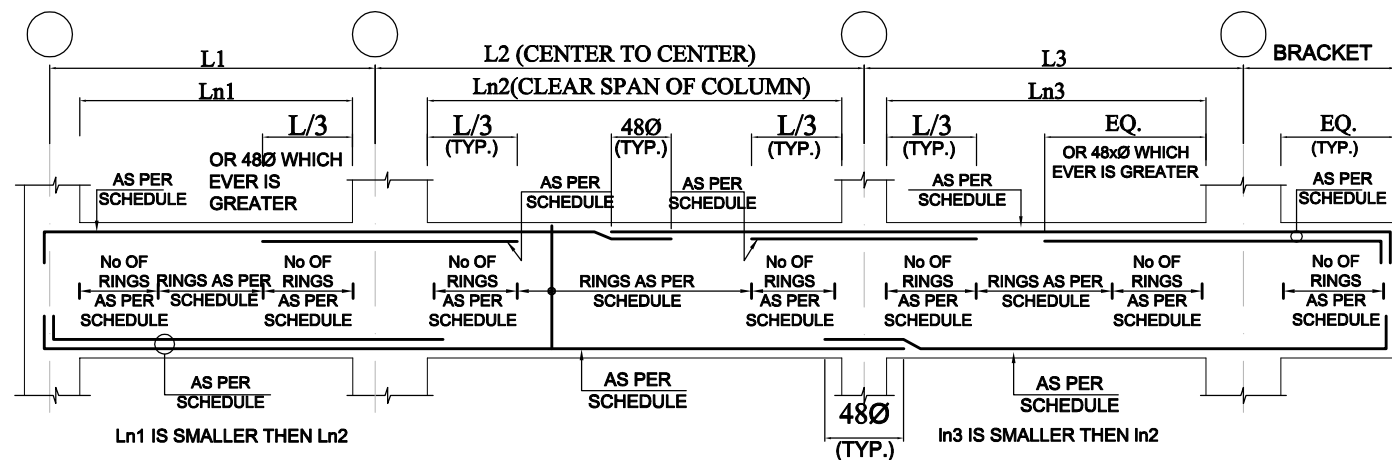
TYP. ELEV. OF PLINTH BEAM
