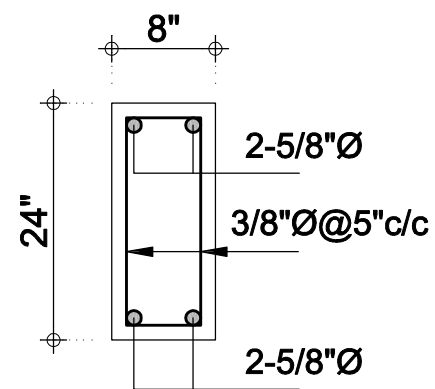
PB-1(8"x24")
