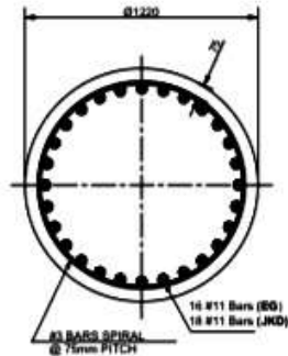
SECTION D-D
