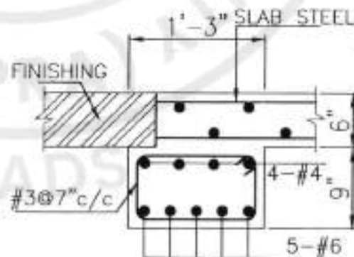
DET-1
