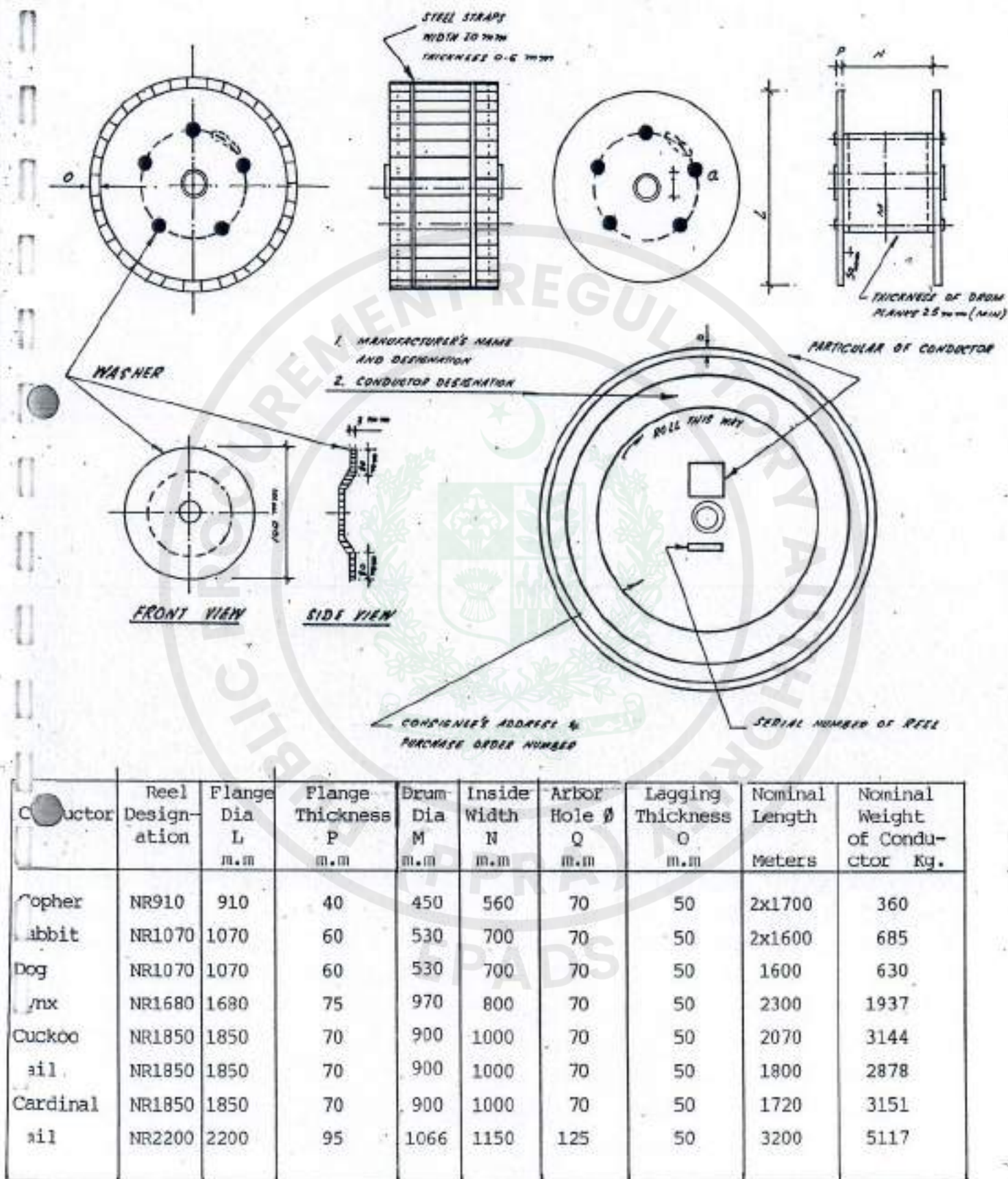
FIG. 1 REEL DIMENSIONS
